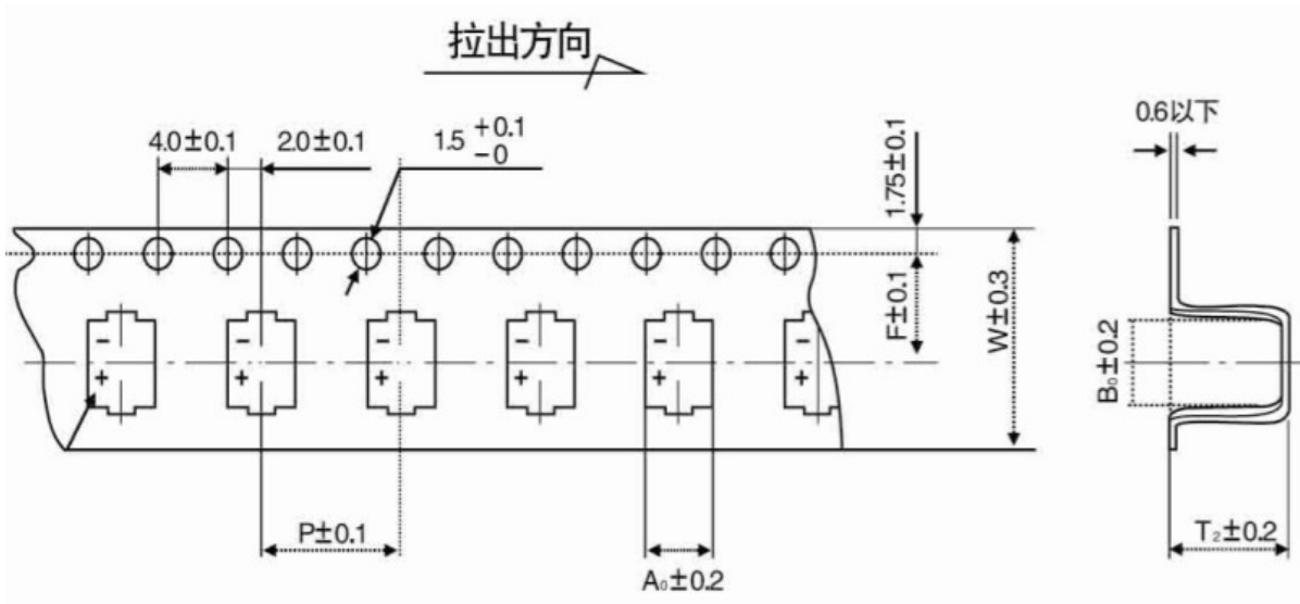
Fig.1 (Ø4 ~ Ø10)
